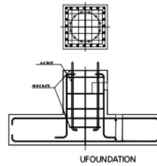
기초방식#2
