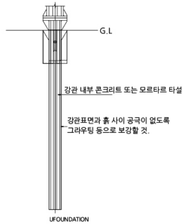
기초방식#1
